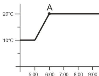
Teplota místnosti: funkce OPTIMUM START zapnuta
