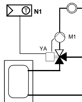
Vybíjení akumulční nádoby směšovaným okruhem
