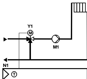
Řízení směšovaného topného okruhu
